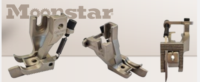
C585 3/16" - B2769 Typical 302-303 Sağ Çima Ön Arka Ayak Takım (4.8mm)
