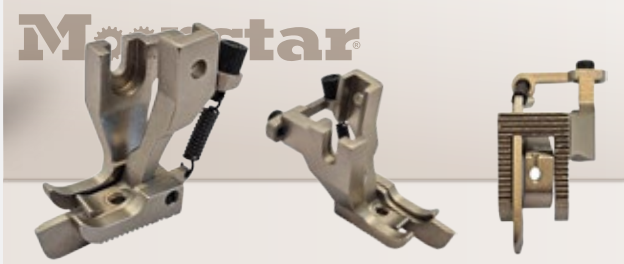
C585 1/8" - B2768 Typical 302-303 Sağ Çima Ön Arka Ayak Takım (3.2mm)
