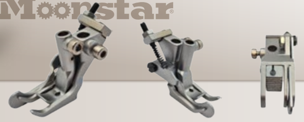
GL867-8 - B2728 Durkopp Adler 367~867 Sol Çima Ön Arka Ayak Takım (8mm)
