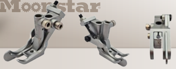
GL867-5 - B2726 Durkopp Adler 367~867 Sol Çima Ön Arka Ayak Takım (5mm)
