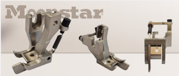
C585 1/4" - B2770 Typical 302-303 Sağ Çima Ön Arka Ayak Takım (6.4 mm)
