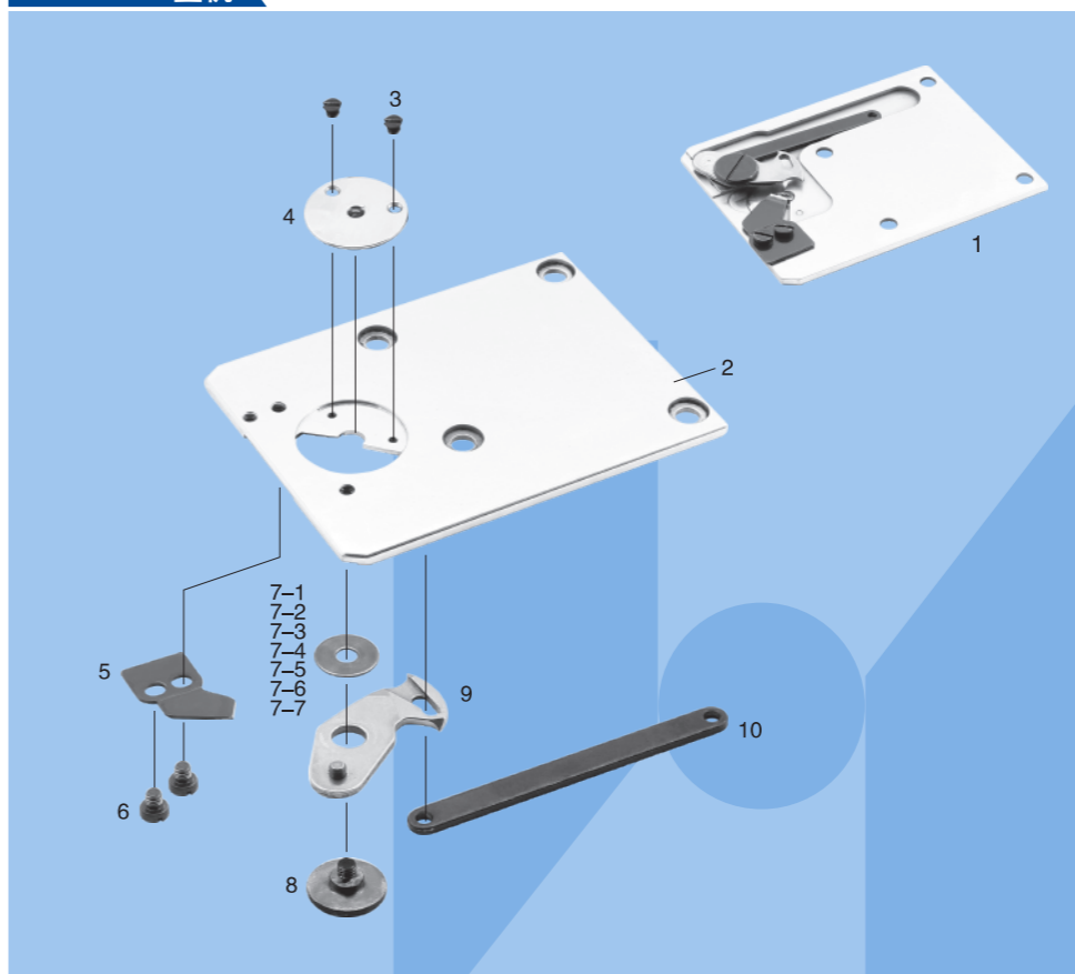
MOL-254 前剪线组件 ASSEMBLY FOR MOL-254
