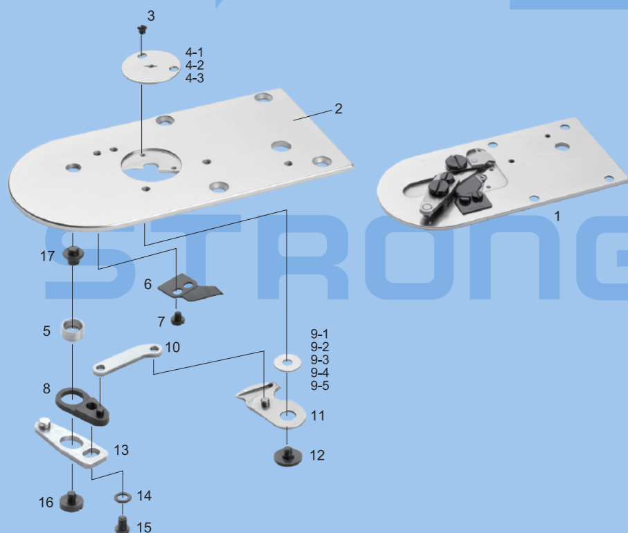
LK-1850 剪线组件 ASSEMBLY FOR LK-1850
