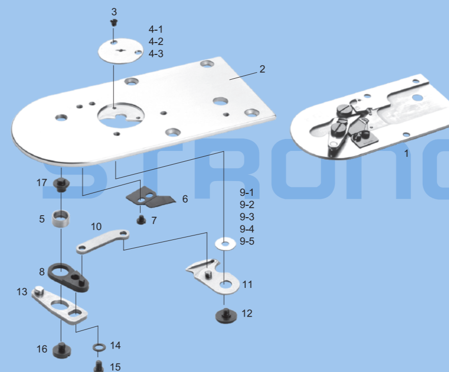
LK-1900A 剪线组件 ASSEMBLY FOR LK-1900A
