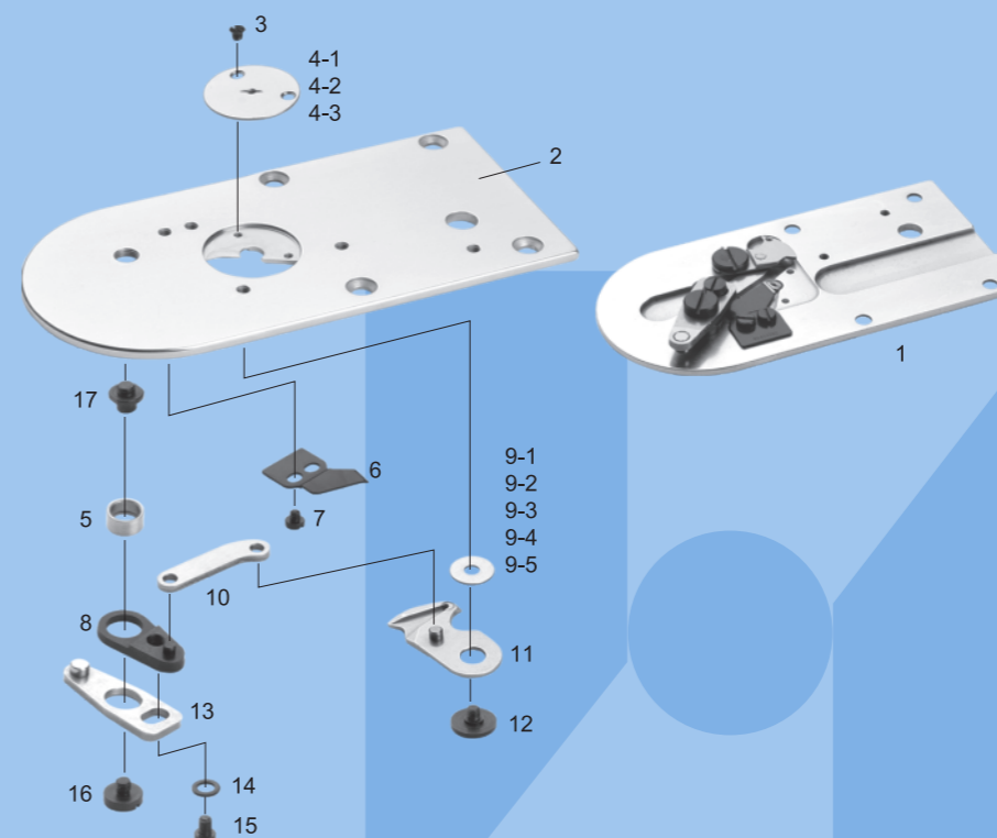
LK-1900 剪线组件 ASSEMBLY FOR LK-1900
