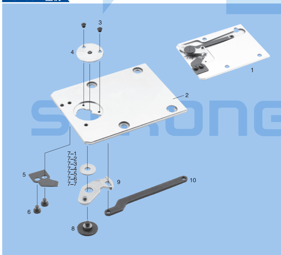
MOL-254 后剪线组件 ASSEMBLY FOR MOL-254
